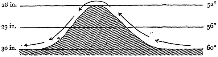
चित्र ३३ : तटस्थ संतुलन (शुष्क वायु के लिये)
